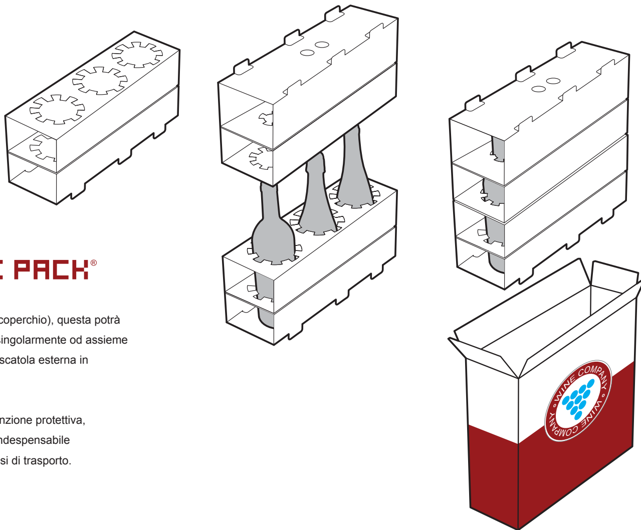
ESEMPIO DI BOX COMPLETO DA 3 BOTTIGLIE CON IMBALLAGGI INTERNI E SCATOLA ESTERNA PERSONALIZZATA
